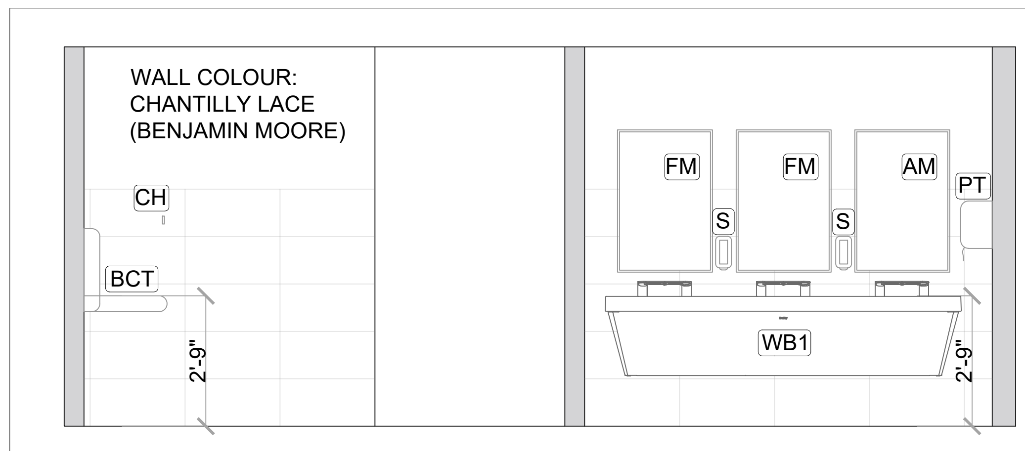
B3170 ELEVATION 4
