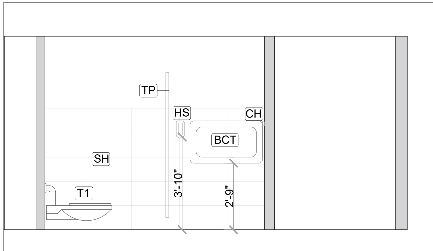
B3170 ELEVATION 1
