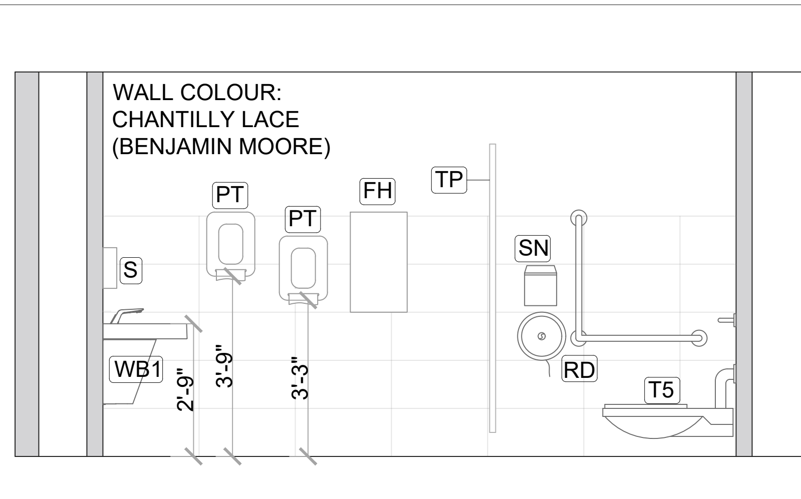
B3170 ELEVATION 2
