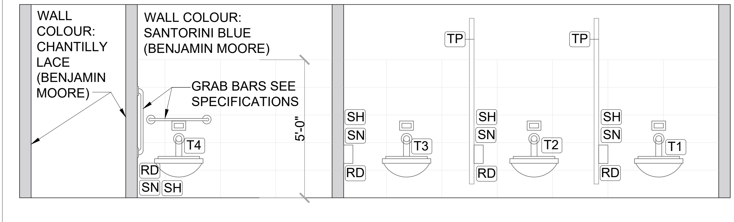
ELEVATION 2
