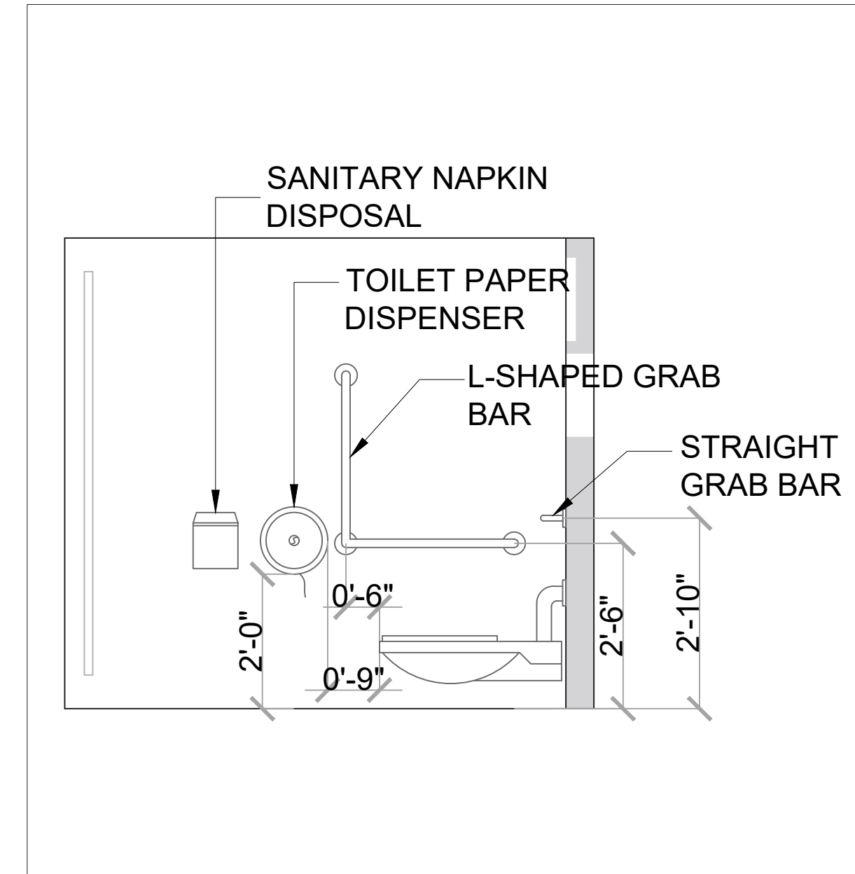
ELEVATION BF2
