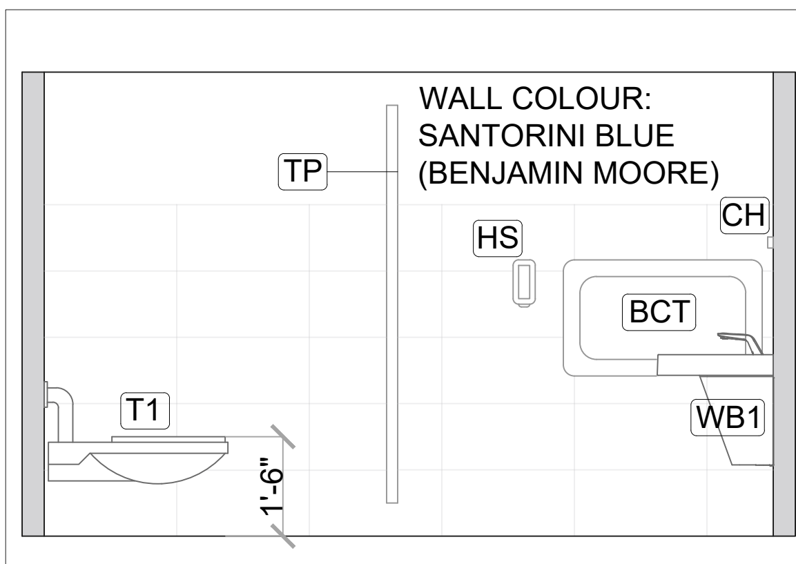
ELEVATION 3
