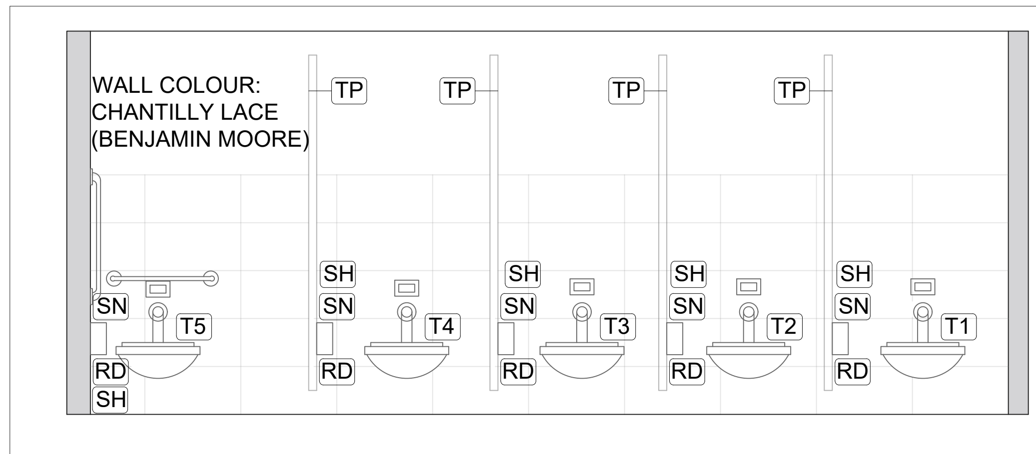
B3170 ELEVATION 3
